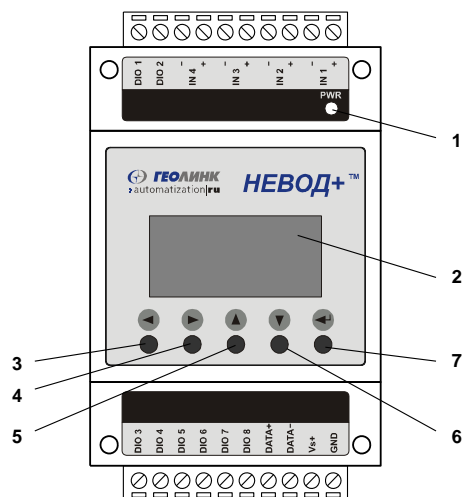
Рис. 3. Расположение элементов управления и индикации на корпусе прибора.
