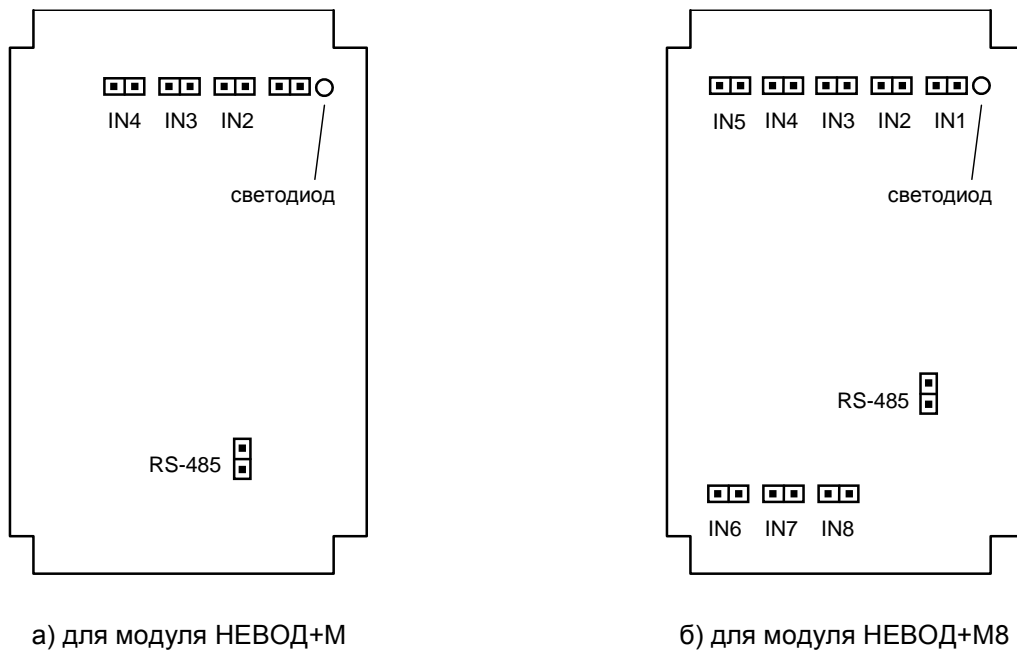
Рис.6. Расположение перемычек на плате прибора.
